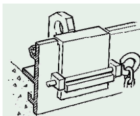
Fig 4b. Paniklås, öppningsbart
