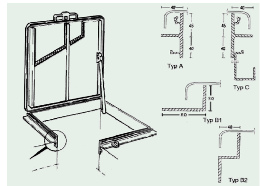
Fig 1. Enkel, överfalsad lucka samt exempel på ramprofiler
