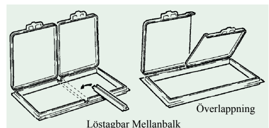
Fig 2. Dubbelluckor, överfalsade med löstagbar mellanbalk resp. överlappning
